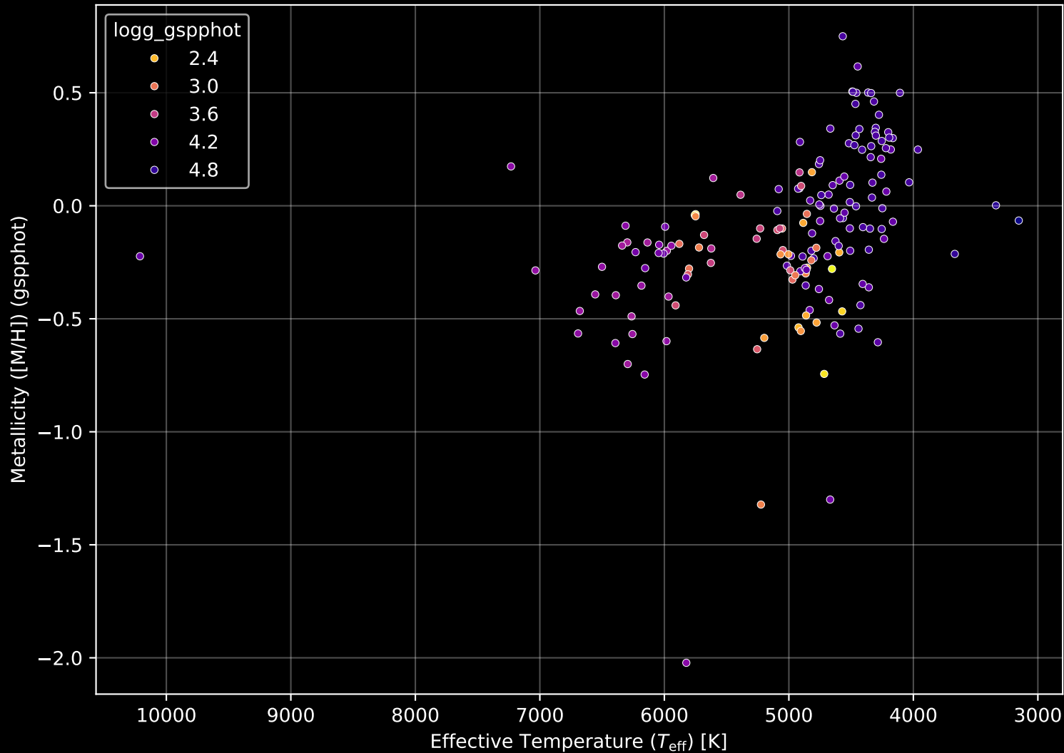
APOGEE DR17 Field: [089+70] Stellar Population Parameters (n= 168)
